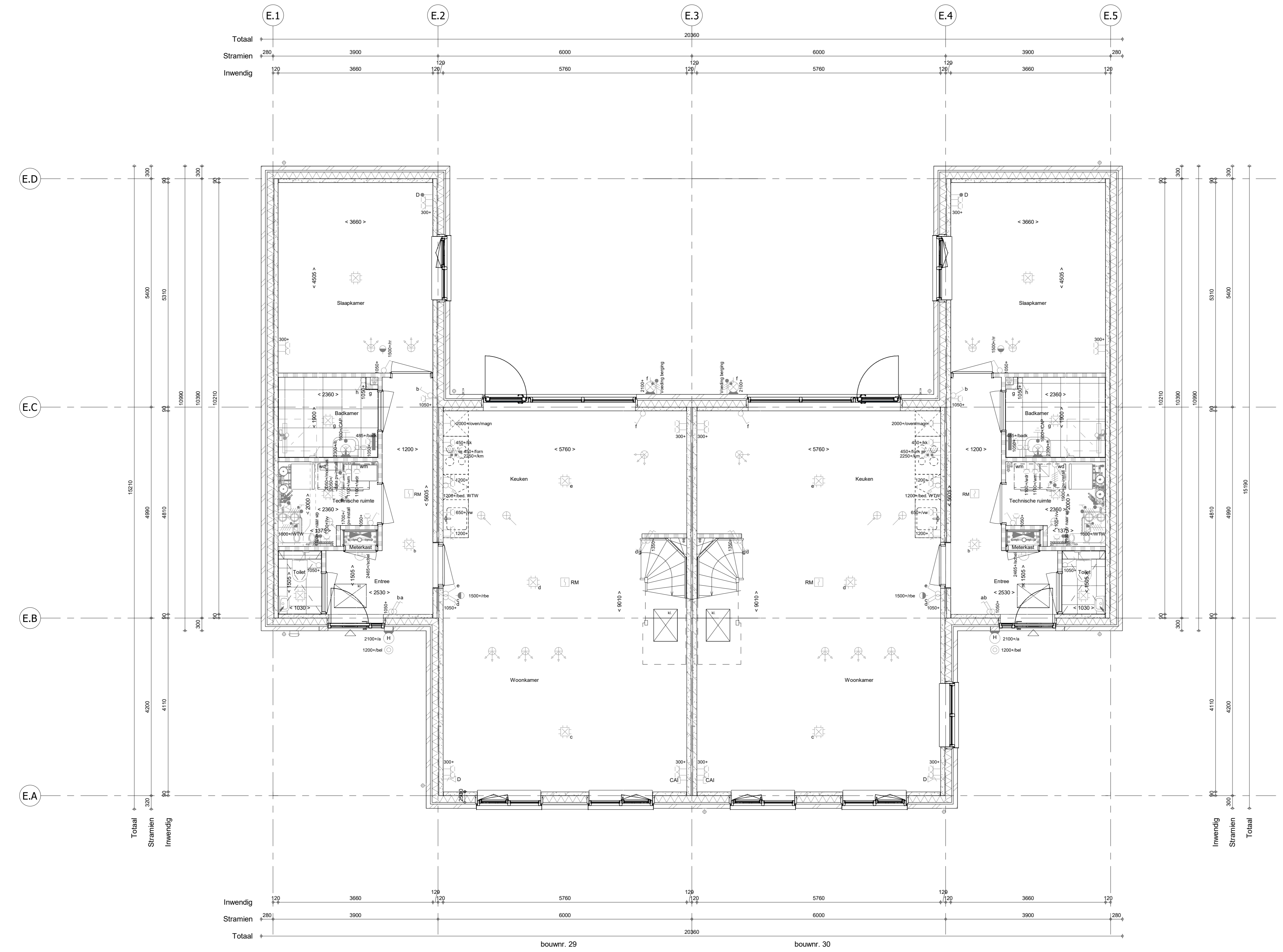
Begane grond 1 : 50
